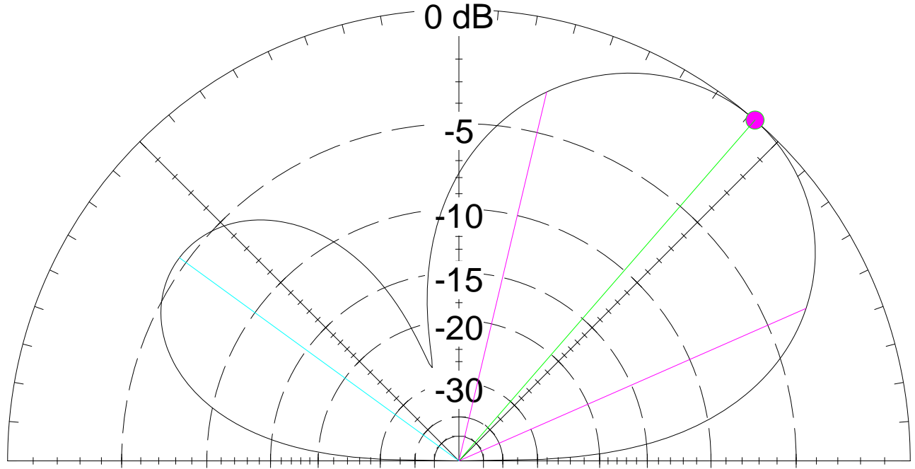
Radio JOVE antenna
