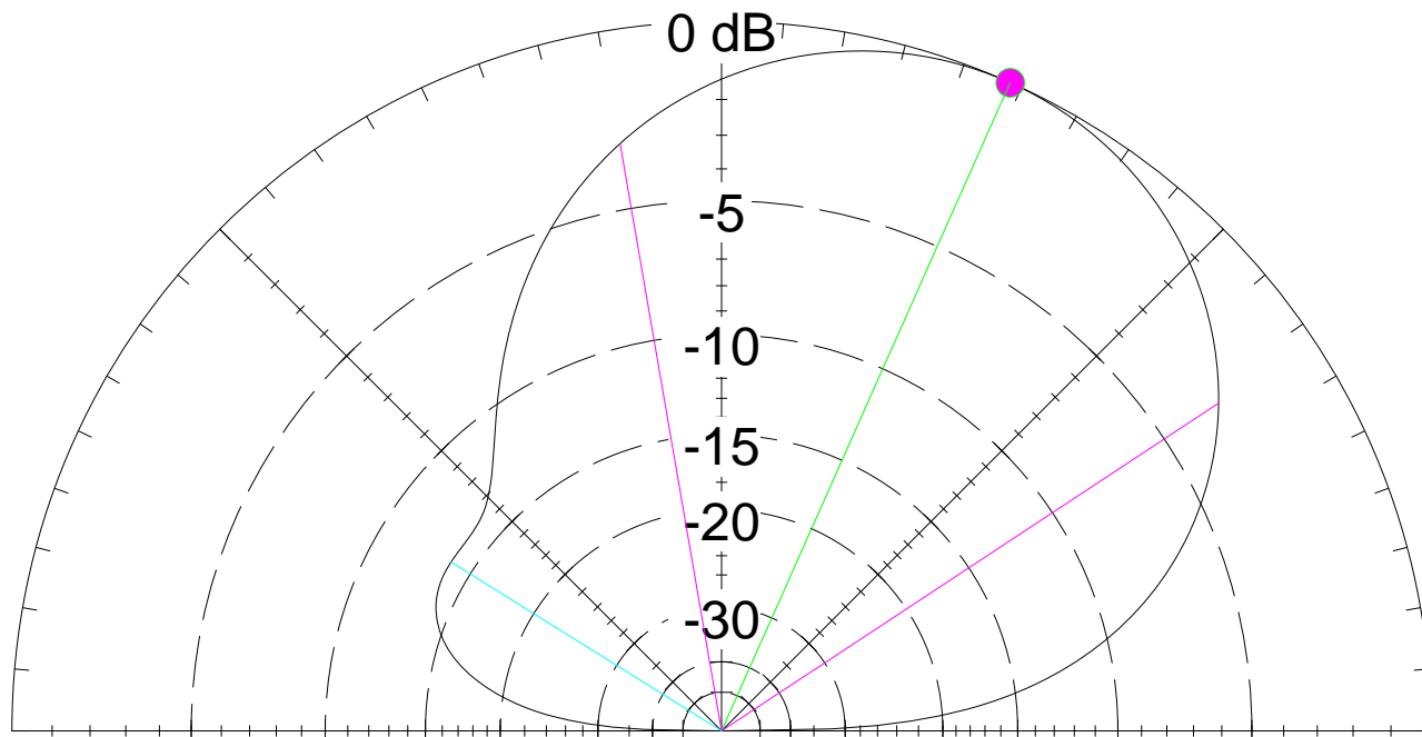
Radio JOVE antenna
