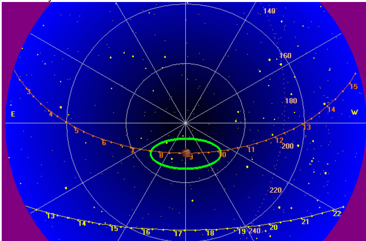
TFD Array 20 MHz HPBW 15° NS x 35° EW
